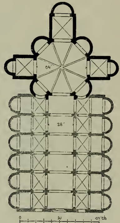
Abb. 116. S. Maria della Passione zu Mailand.
